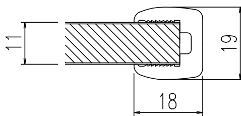
A-A'断面 (1/1)
