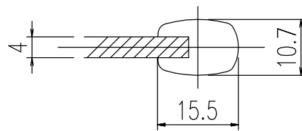
A-A 断面図 (S=1/1)
