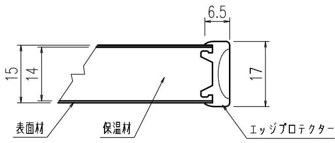
A-A 断面図 (S=1/1)
