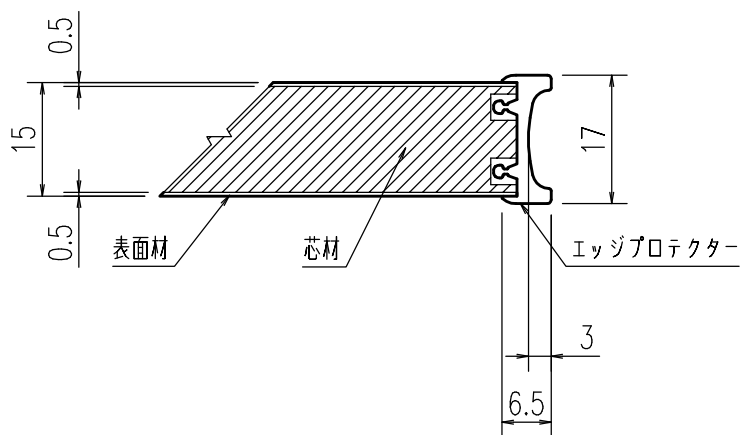
A-A断面図 (S=1/1)
