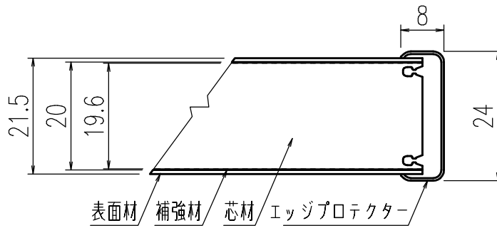
A-A断面図 (S=1/1)
