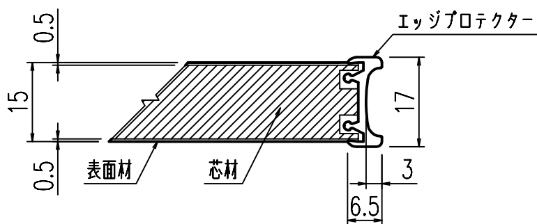
A-A断面図 (S=1/1)
