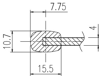
A-A断面(S=1/1)
