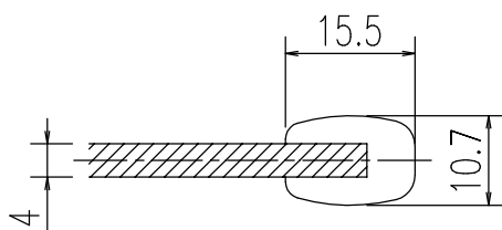
A-A断面 (S=1/1)
