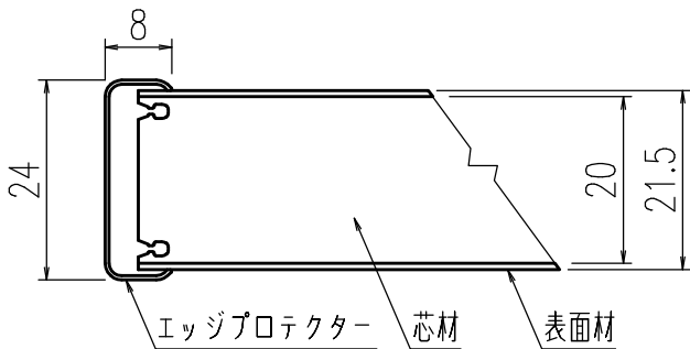
B-B断面図 (S=1/1)
