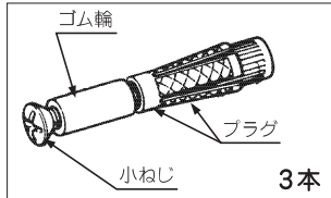
AYボルト仕様
