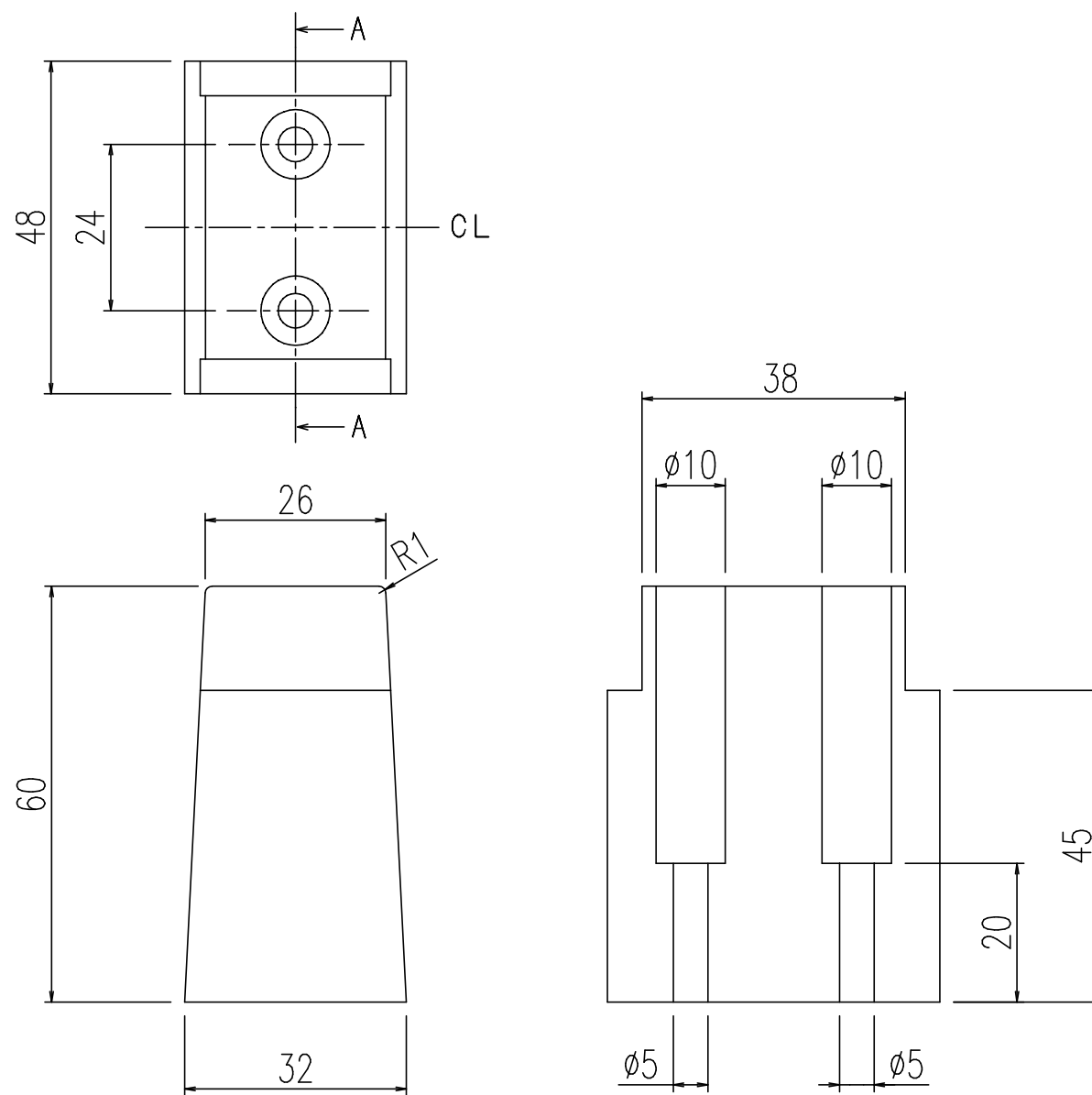
A-A断面
