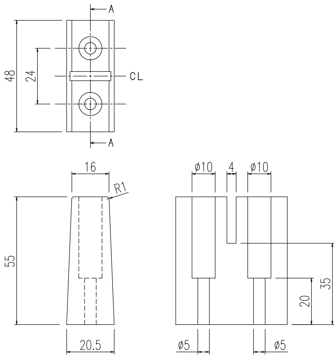
A-A断面
