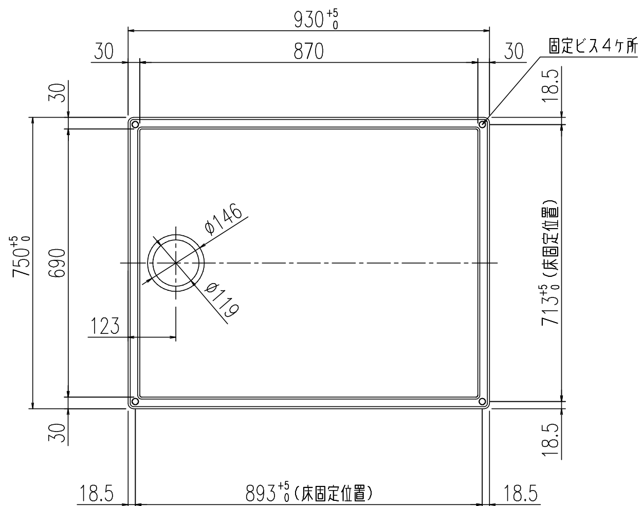
PFL-100/FW1 (φ6 L=100 4本, 化粧キャップ付)
