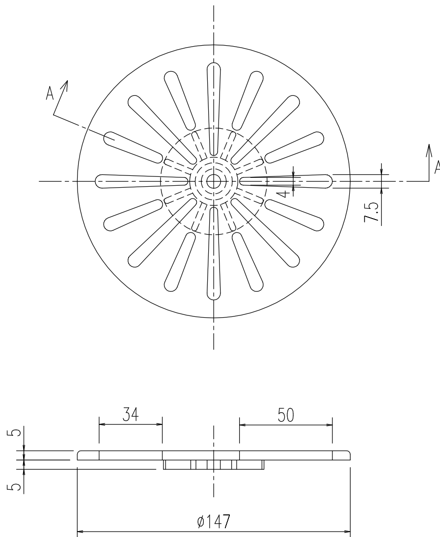
A-A 断面
