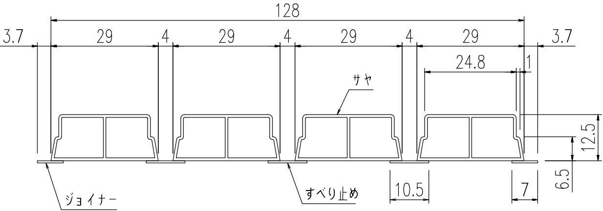
A-A' 断面図 (S=1/1)
